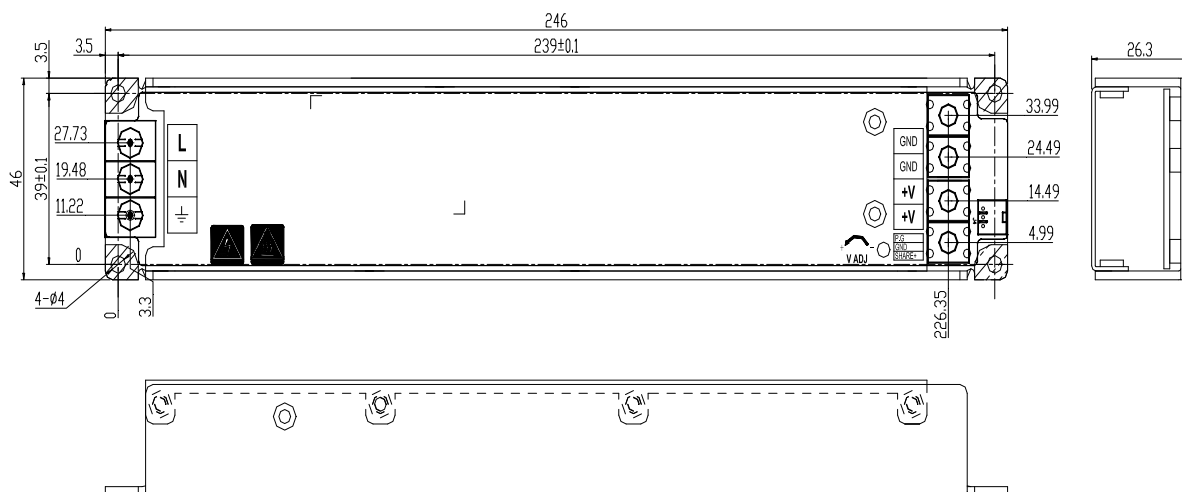
外形尺寸及安装孔——端子坐标图
